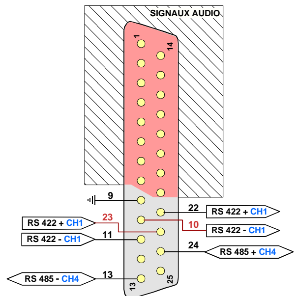
Connecteur DB 25 femelle (ERC AD) 1 RS 422 1 RS 485 2 fils
