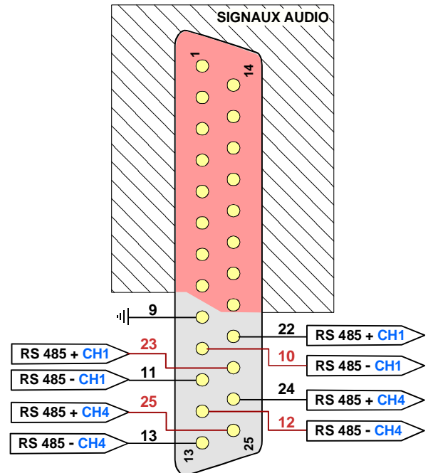
Connecteur DB 25 femelle (ERC AD) 2 RS 485 4 fils
