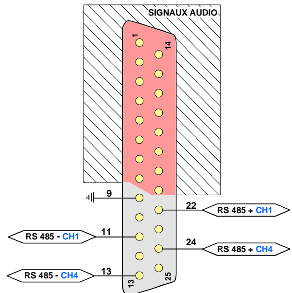
Connecteur DB 25 femelle (ERC AD) 2 RS 485 2 fils
