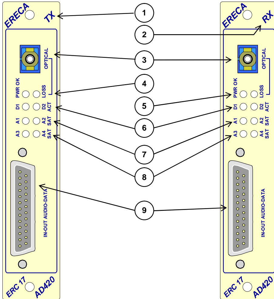
Figure 2 : Face avant des modules ERC AD 420
