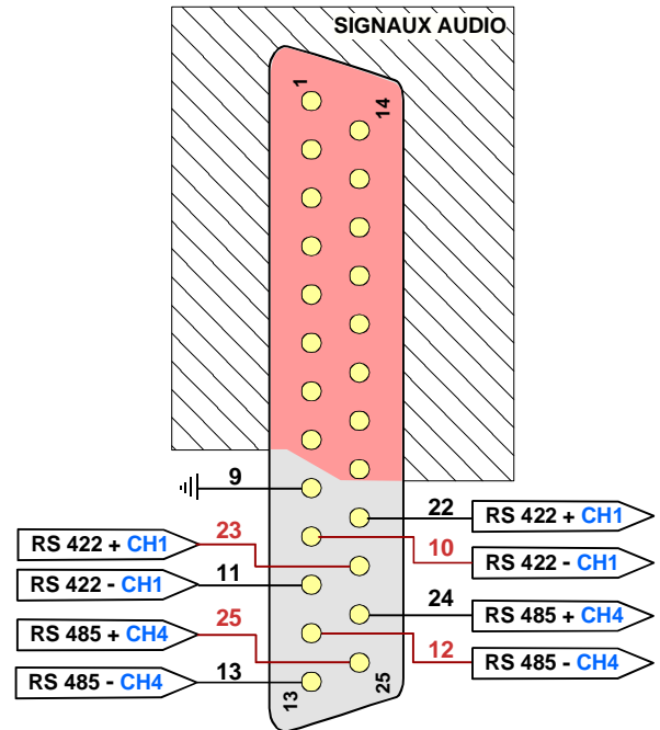
Connecteur DB 25 femelle (ERC AD) 1 RS 422 1 RS 485 4 fils
