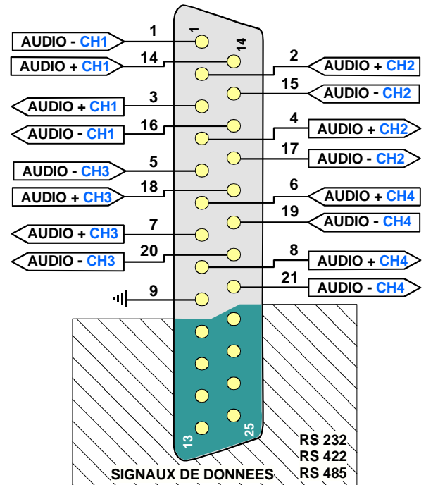
Connecteur DB 25 femelle (ERC AD) 4 voies audio bidirectionnelles
